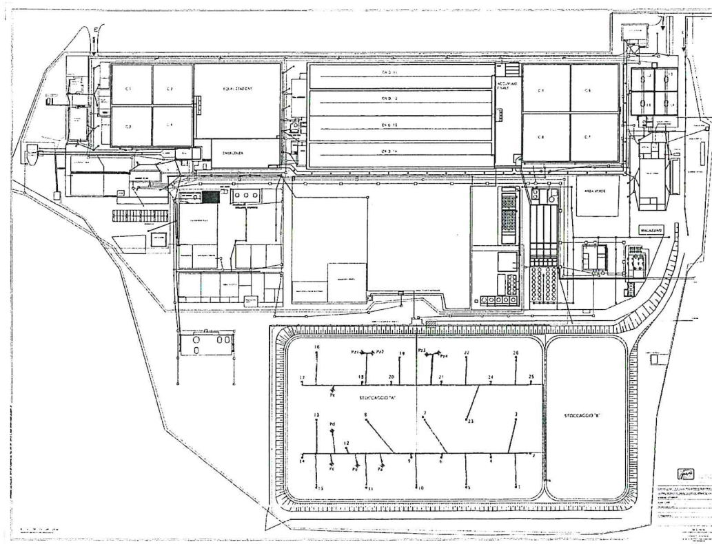
Assieme interrati
